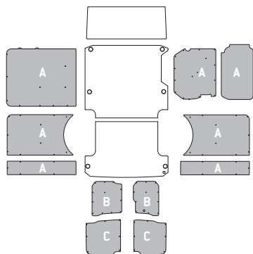
Fahrzeugtyp - Model L1 H1 · 3000 H1 A
