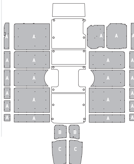
Fahrzeugtyp - Model L3L H3 · 4100L H3 B
