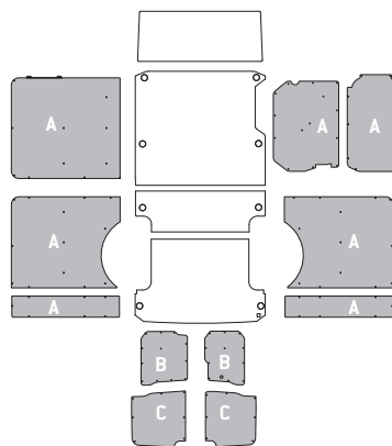
Fahrzeugtyp - Model L2L H3 · 3520L H3 A
